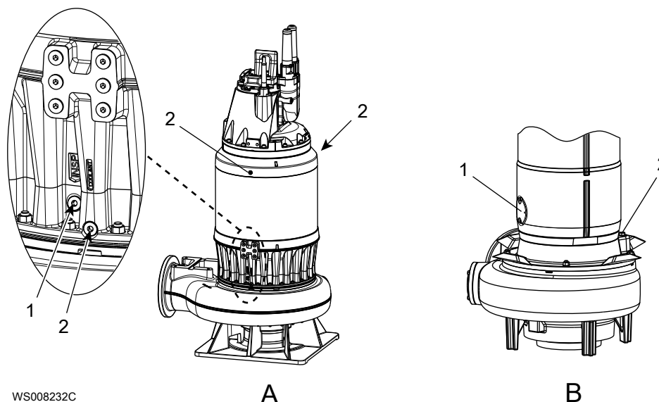
Рис. 75: А: блок привода с рубашкой охлаждения. В: блок привода без рубашки охлаждения.
