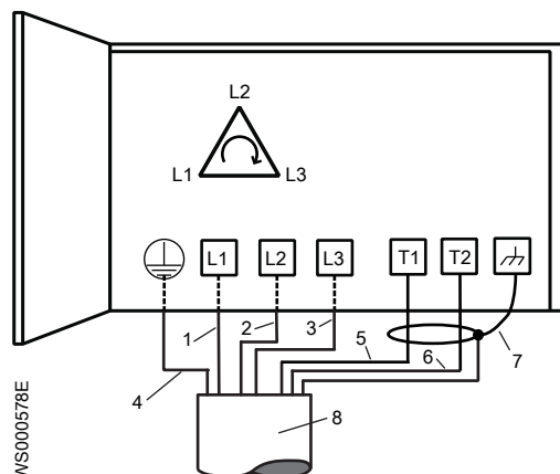
Рис. 56: Правильное чередование фаз
