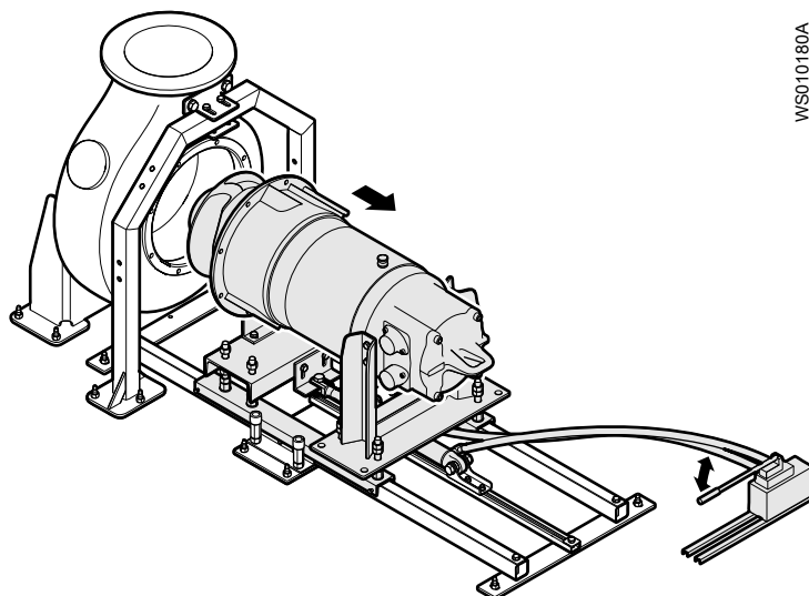
Рис. 87: Передвижение блока привода при помощи ручного насоса
