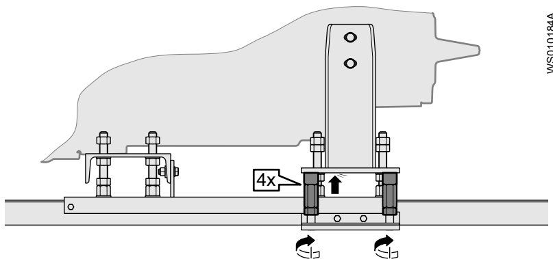
Рис. 94: Подъем внешних опор
