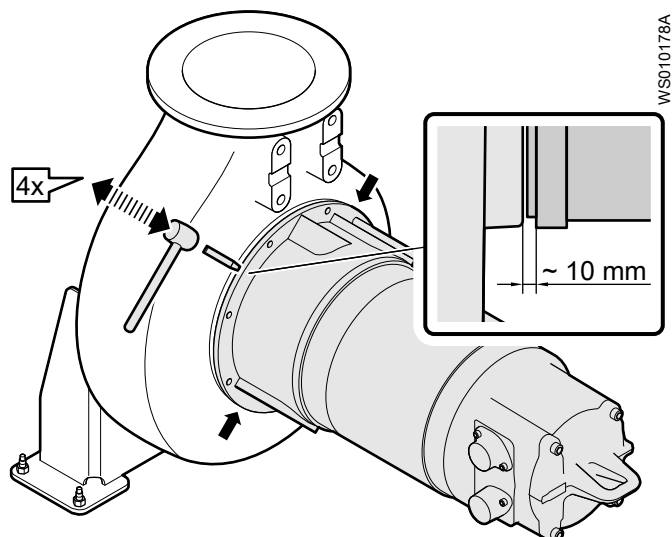
Рис. 85: Демонтаж блока привода
