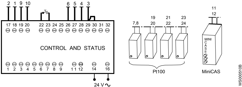
Рис. 55: Подключения к основному блоку CAS.
