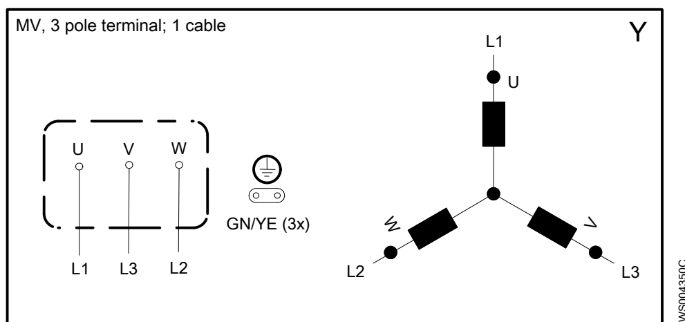
Рис. 61: Схема обмотки для блоков приводов со средним напряжением (1,2 – 6,6 кВ)
