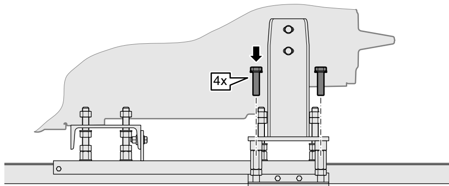
Рис. 96: Вставка болтов внешних опор
