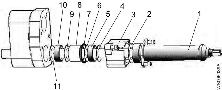
Рис. 47: Блоки привода 605-776
