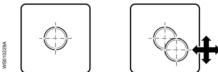
Рис. 89: Совмещение отверстий блока привода со шпильками корпуса насоса
