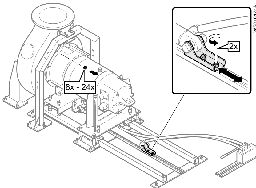
Рис. 81: Подготовка блока привода к перемещению
