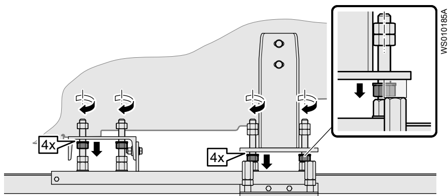
Рис. 95: Перемещение гаек вниз под обеими опорными плитами
