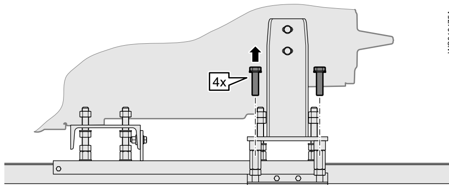
Рис. 82: Снятие болтов
