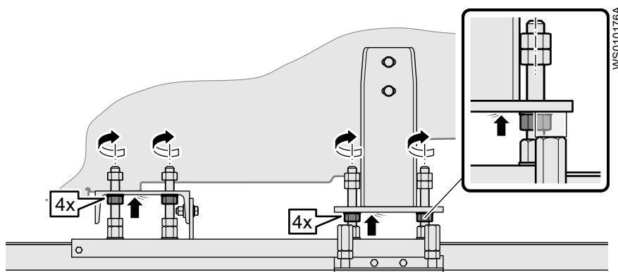
Рис. 83: Перемещение гаек вверх под обеими опорными плитами
