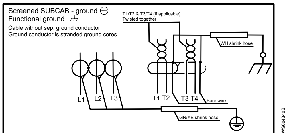
Рис. 59: Без отдельного провода заземления.
