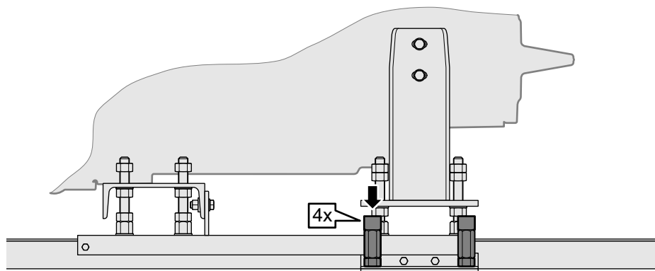
Рис. 84: Опускание внешних опор
