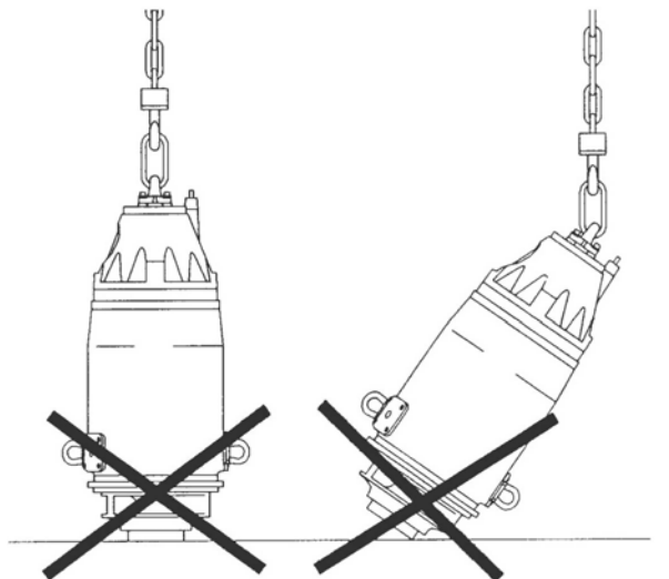
Рис. 77: Неправильный способ подъема
