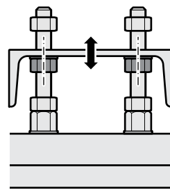
Рис. 91: Регулировка по вертикали
