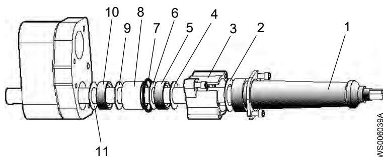
Рис. 45: Блоки привода 605-776
