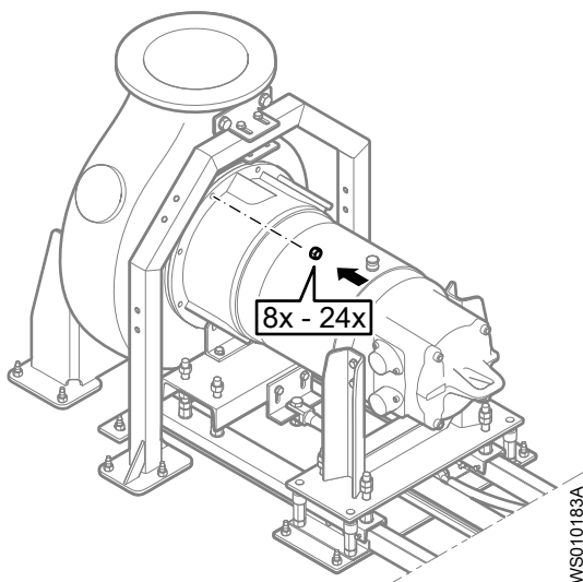
Рис. 93: Крепление блока привода к гидравлическому блоку
