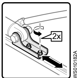
Рис. 92: Ослабление гаек поршня
