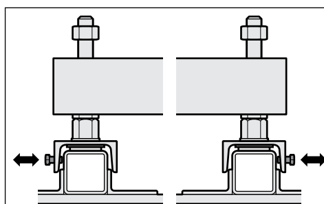
Рис. 90: Регулировка по горизонтали
