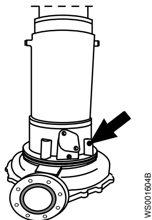
Рис. 62: Вход для линии подачи охлаждающей жидкости
