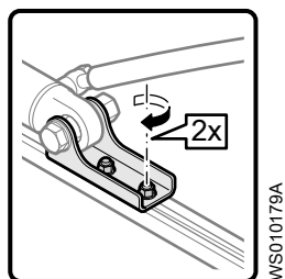
Рис. 86: Затяжка гаек поршня ручного насоса
