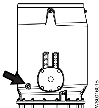
Рис. 64: Вход для линии подачи охлаждающей жидкости
