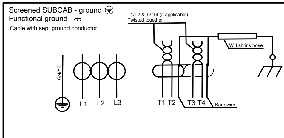
Рис. 60: С действующим заземлением
