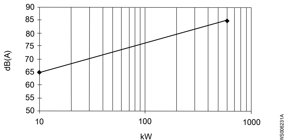
Рис. 68: Звуковое давление
