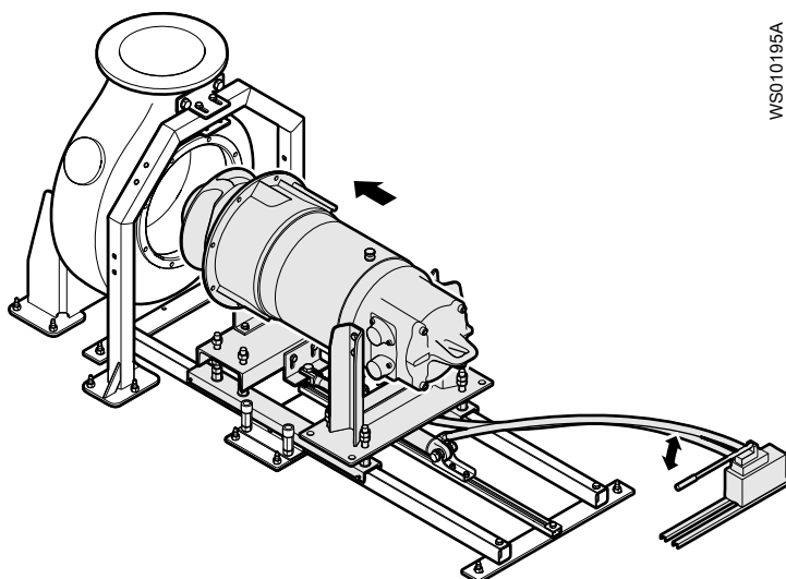
Рис. 88: Передвижение блока привода при помощи ручного насоса
