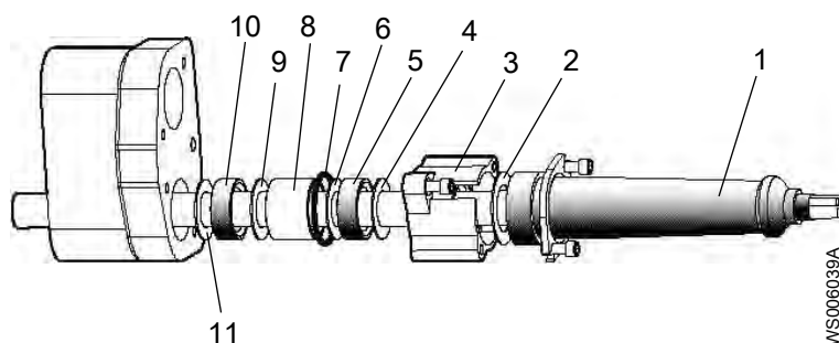
Рис. 49: Блоки привода 605-776
