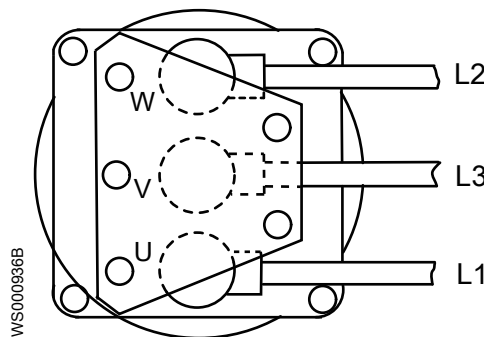
Рис. 61: Схема обмотки для блоков приводов со средним напряжением (1,2 – 6,6 кВ)
